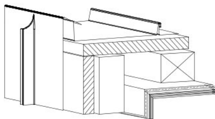
Detal: połączenie elewacji na rąbek z dachem
