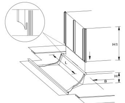
Detal: przykładowa obróbka komin
