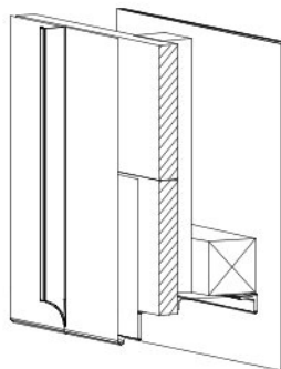
Detal: zakończenie elewacji na rąbek
